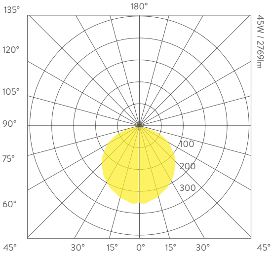
ZIRKOL CEILING
