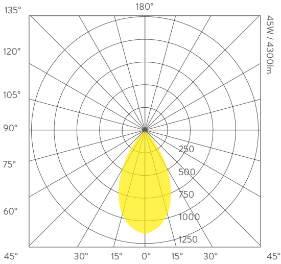
LINEAR UGR
