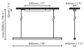
BLOKINLINE LEDTUBE S 900
