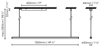
BLOKINLINE LEDTUBE S 1200
