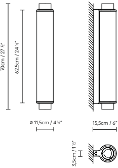
SLIM SKIN W700
