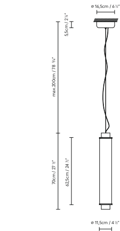
SLIM SKIN SV 700
