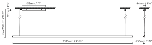
BLOKINLINE LEDTUBE S 2400
