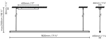
BLOKINLINE LEDTUBE S 1800
