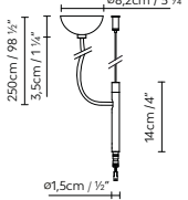
KUPETZ SINGLE SUSPENSIÓN
