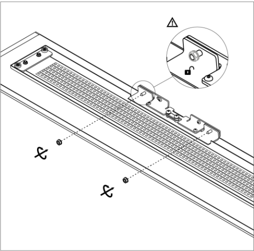
Adjustement B
