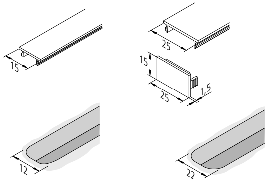
Abdeckung der Fräsnut oder für Alu-Profile
