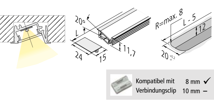
Innenliegendes asymmetrisches Profil für LED Streifen
