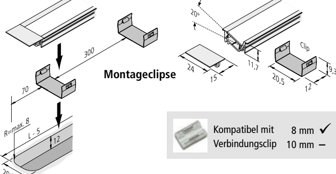
Clipbares, asymmetrisches Profil für LED Streifen
