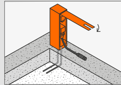
jack . Steckdosensäule jack . connecting pillar
