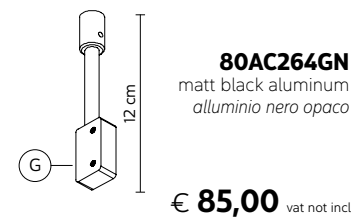
bar hook h12 - gancio per barra
