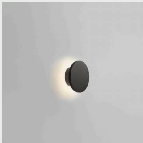
SOHO W1 / EURO 222,- EX VAT / SEK 2.420,- EX VAT 6W LED - IP54 - 2700/3000K - CRI >90 Black - 270144 Ø120 mm
