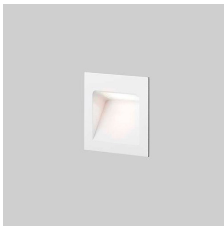
DELI 1 / EURO 188,- EX VAT / SEK 2.060,- EX VAT 4,5W LED - IP54 - 3000K - CRI >90 White - 260880 90x90 mm
