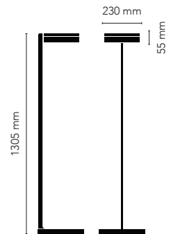
BLADE F1 SLIM 12.5W LED - 220-240V Page 32
