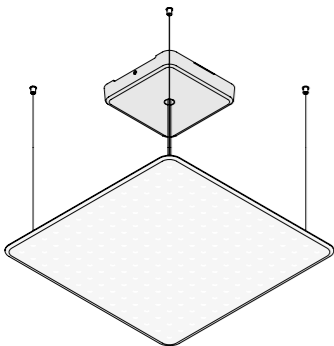
MODUL Q 600 PROJECT Pendelleuchte / Suspended luminaire
