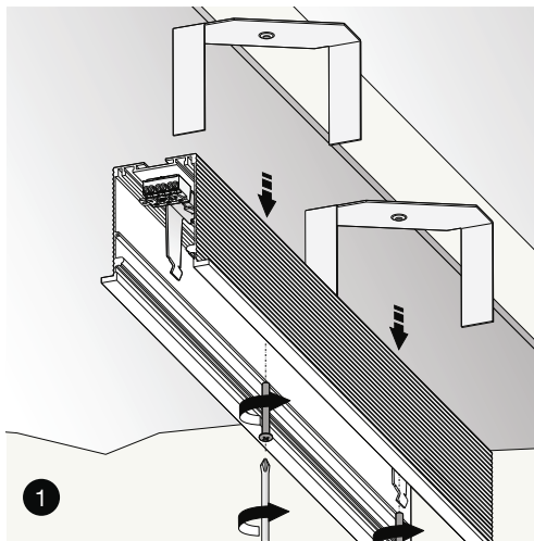
XM2038/39-U Giunzione lineare Linear junction
