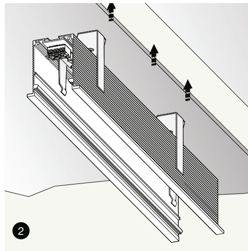
XM2038/39-ANG Giunzione 90° trim parete-soffitto 90° wall to ceiling trim junction
