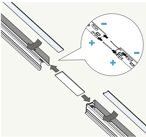
XM2033/34-U Giunzione lineare Linear junction
