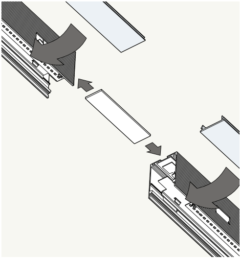
XG2038-U90 Giunzione piana 90° trimless con LED e driver Level junction 90° trimless with LED and driver
