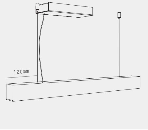
PENDANT / Power box model
